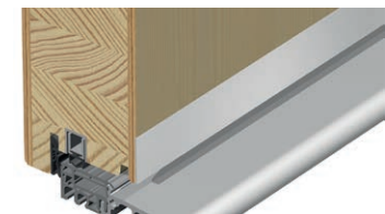
Trittschutzblech W2 Edelstahlblech 25 mm, flächenbündig Optional schwarz lackiert W2B
