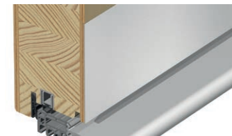
Trittschutzblech W7 Edelstahlblech 85 mm, flächenbündig Optional schwarz lackiert W7B
