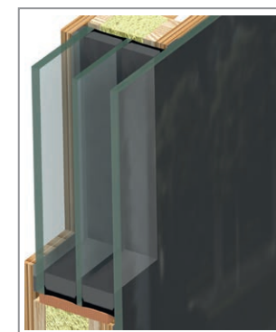
3-fach Verglasung mit Email Außen Klarglas oder Parsol grau mit email schwarz / mittig Klarglas oder Satinato weiß / innen Klarglas Holz & Holz-Alu Serie VETRO
