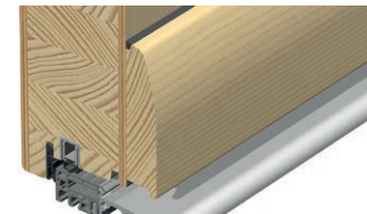
Wetterschenkel W1 Holzprofil 85 mm
