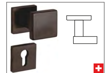
G5S Feststehender Knopf - VERSETZT Edelstahl schwarz matt
