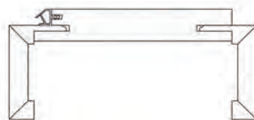
G65-T30 Brandschutzzarge 65 mm Bekleidung eckig, ohne Profil Bekleidungen auf Gehrung
