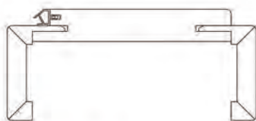
R65 Normzarge rund 65 mm Bekleidung rund, ohne Profil Bekleidungen auf Gehrung (nicht in Eiche astig)
