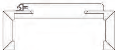
Furnierte Softzarge FR 60 mm Bekleidung abgerundet R2, ohne Profil Bekleidungen auf Gehrung
