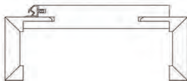
Furnierte Softzarge FE 60 mm Bekleidung eckig, ohne Profil Bekleidungen auf Gehrung
